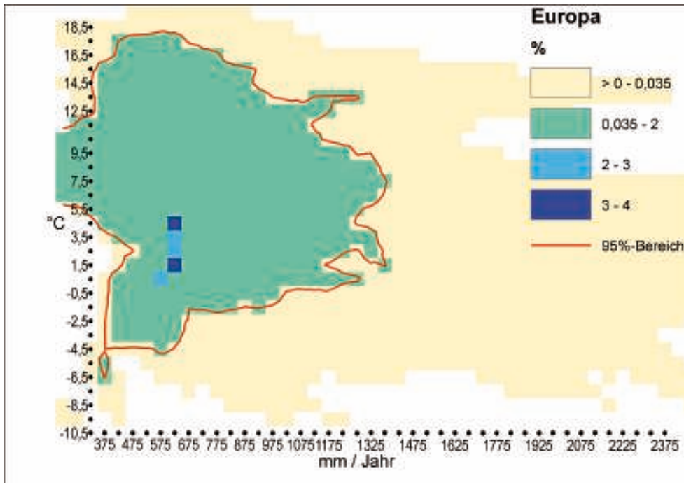
Bild 5. Klimahülle für Europa (trockenste Bereiche nicht dargestellt)
