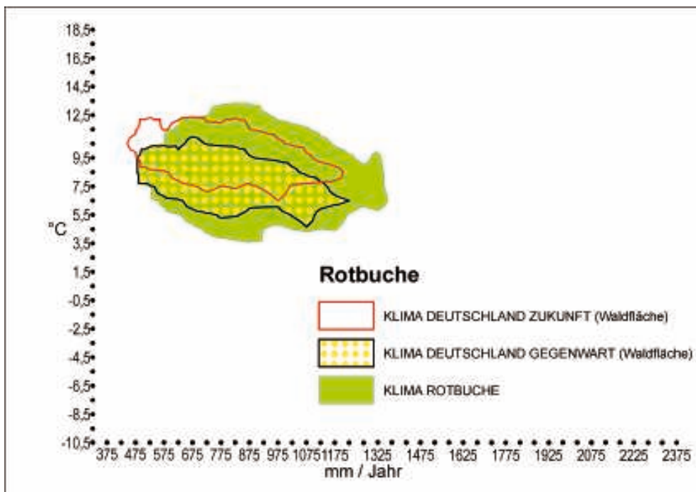
Bild 9. Klimahülle einer Baumart mit mitteleuropäischer Verbreitung (Rotbuche) im Vergleich mit der gegenwärtigen und einer möglichen zukünftigen Klimahülle von Deutschland.
