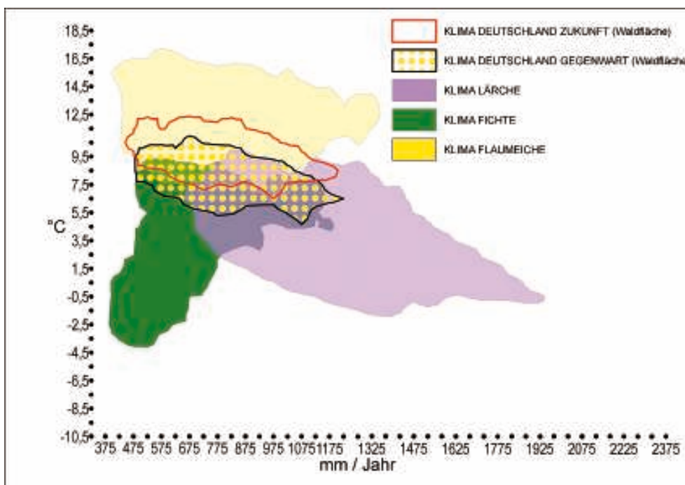
Bild 10. Klimahüllen von Baumarten mit borealer (Fichte), alpischer (Lärche) und submediterranean (Flaumeiche), Verbreitung im Vergleich mit der gegenwärtigen und einer möglichen zukünftigen Klimahülle von Deutschland.
