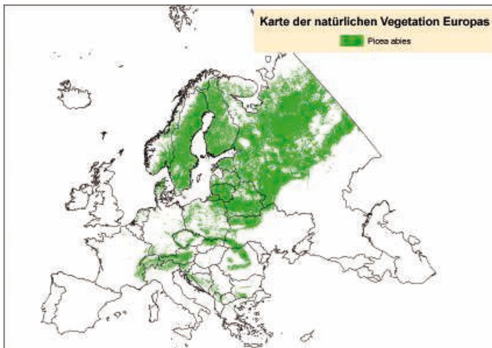
Bild 3. Verbreitungsgebiet der boreal-alpinen Baumart Fichte [13].
