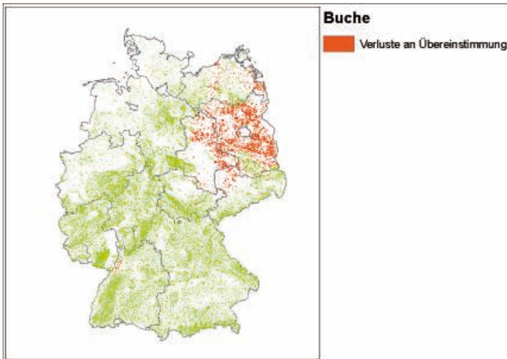
Bild 12. Kartendarstellung der Verluste an Übereinstimmung der Klimahüllen von Rotbuche und Deutschland beim angenommenen Klimaszenario (vgl. Bild 9).
