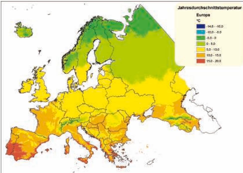
Bild 1. Gegenwärtige (1950 bis 2000) Jahresmitteltemperaturen in Europa [12].
