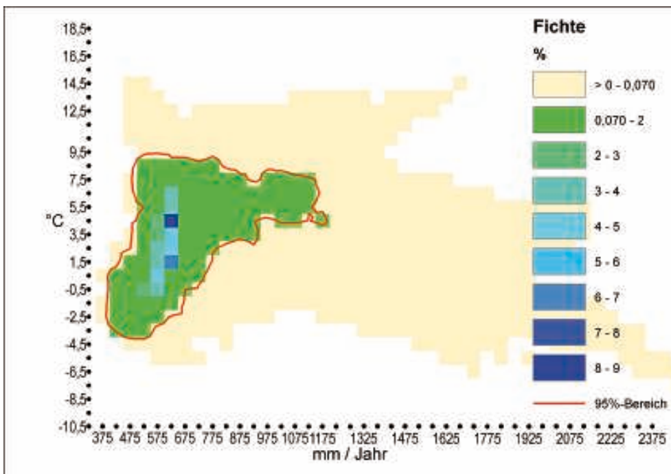
Bild 6. Klimahülle der Baumart Fichte.
