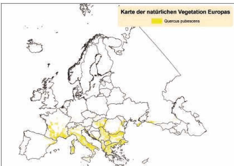
Bild 4. Verbreitungsgebiet der submediterranen Baumart Flaumeiche [13].
