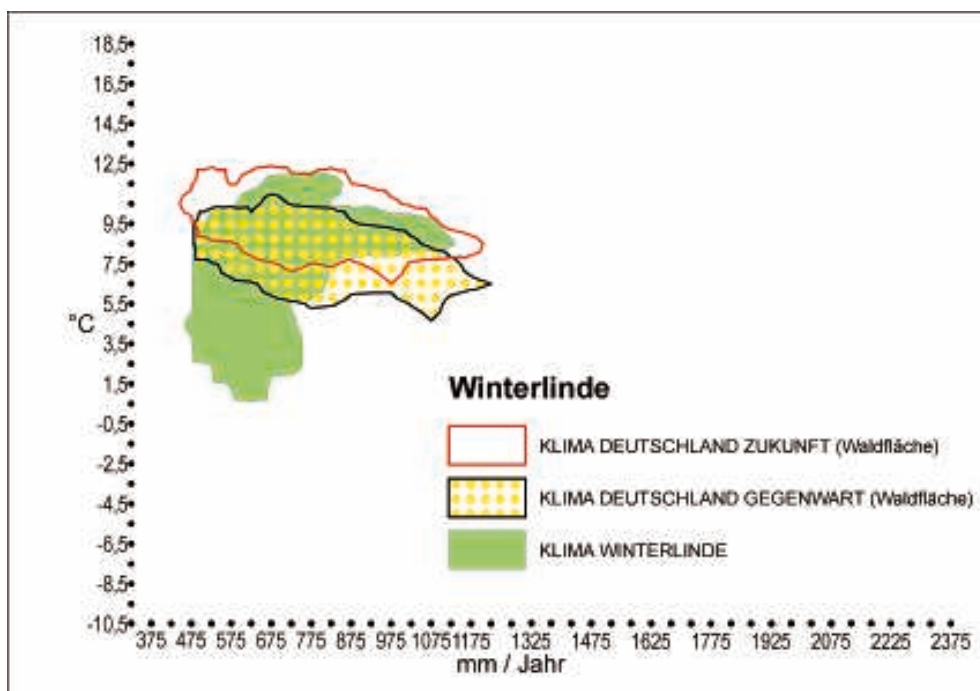
Bild 11. Klimahülle der Winterlinde im Vergleich mit der gegenwärtigen und einer möglichen zukünftigen Klimahülle von Deutschland. In bislang kühl-feuchten Regionen kommt es zur Mehrung der Übereinstimmung von 17 %, in den warm-trockenen Regionen zu einer Minderung um 27 %. Netto sinkt die Übereinstimmung in Deutschland um 10 %.
